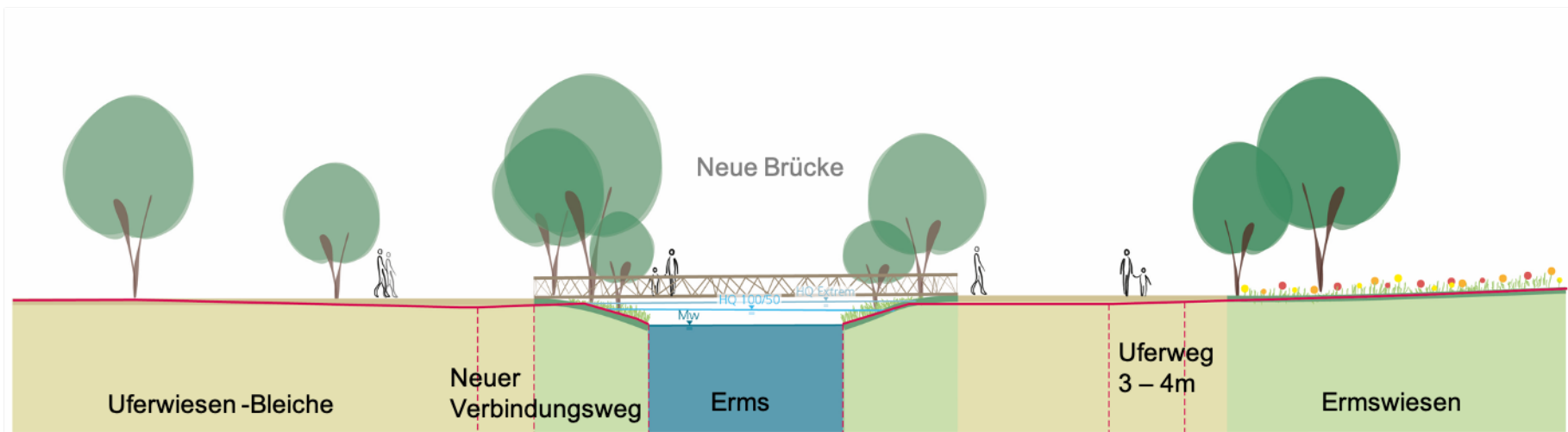
Schnitt 9 Bleiche - neue Brücke
